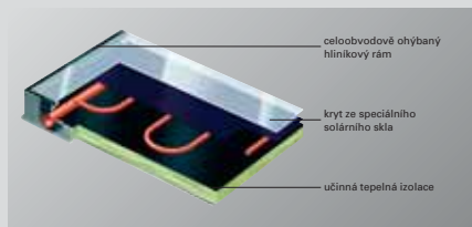
Vitosol 100-F v řezu
